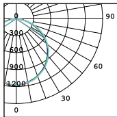
CBO-LED-231 36W
