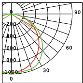
CBO-LED-231 48W
